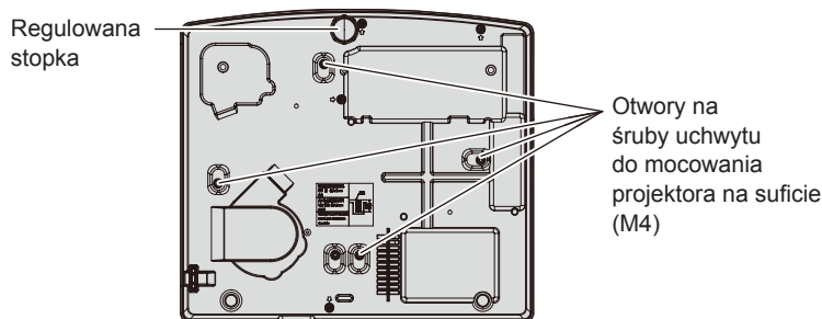
Położenie gwintowanych otworów do montażu uchwytu do mocowania na suficie oraz regulowana stopka
