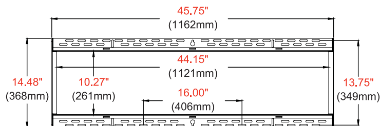
SZCZEGÓŁY PŁYTY ŚCIENNEJ
